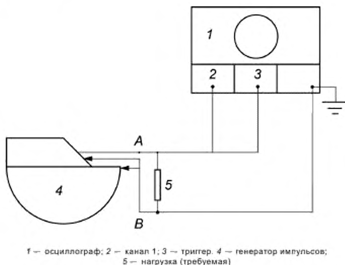
Рисунок 101 — Испытательная установка для измерения характеристик импульса стимуляции
