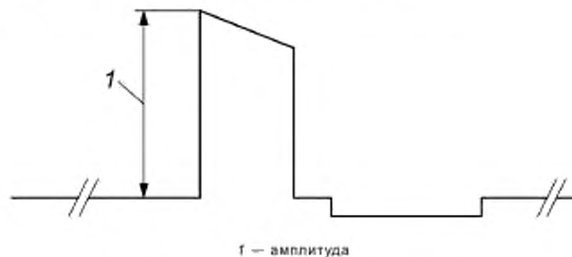
Рисунок 102 — Измерение амплитуды импульса
