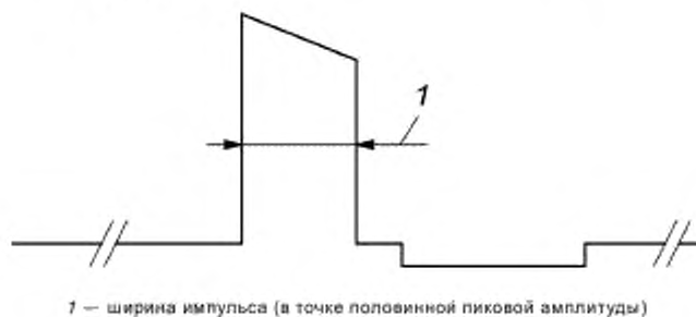
Рисунок 103 — Измерение ширины импульса
