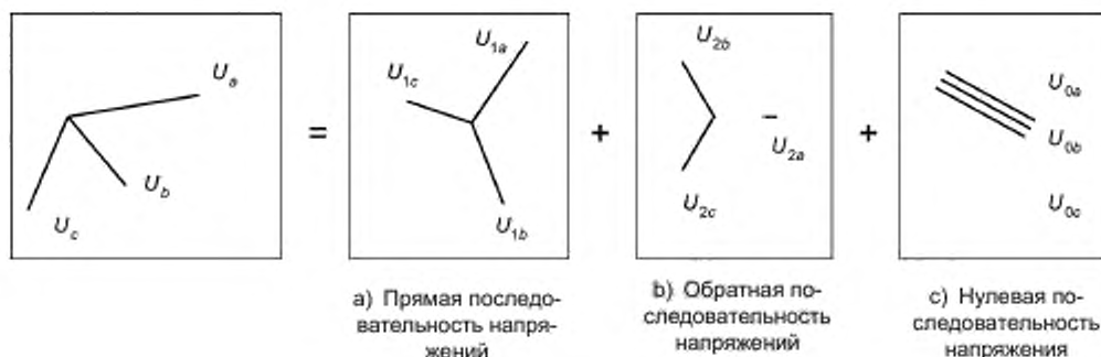
Рисунок А.2 — Составляющие несимметричных векторов на рисунке А.1
