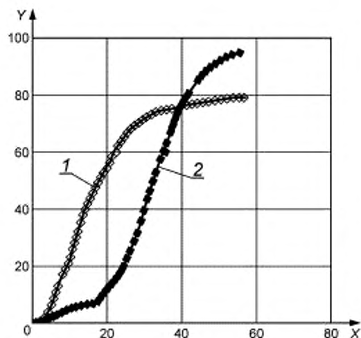
Рисунок А.5 — Результаты испытания на биоразложение порошка ПМК [средний размер частиц — (214,2 \pm 64,7) мкм] в процессе контролируемого компостирования при 58^{\circ}\text{C} в соответствии с ГОСТ Р 57219 (в качестве контрольного материала использовали порошок целлюлозы с размером частиц менее 20 мкм)
