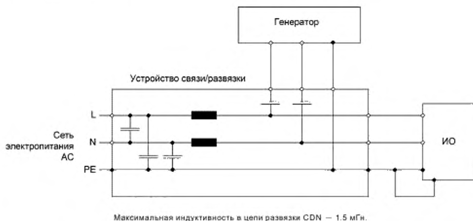
Рисунок 9b — Испытательная установка, снабженная специальными заземляющими проводниками
