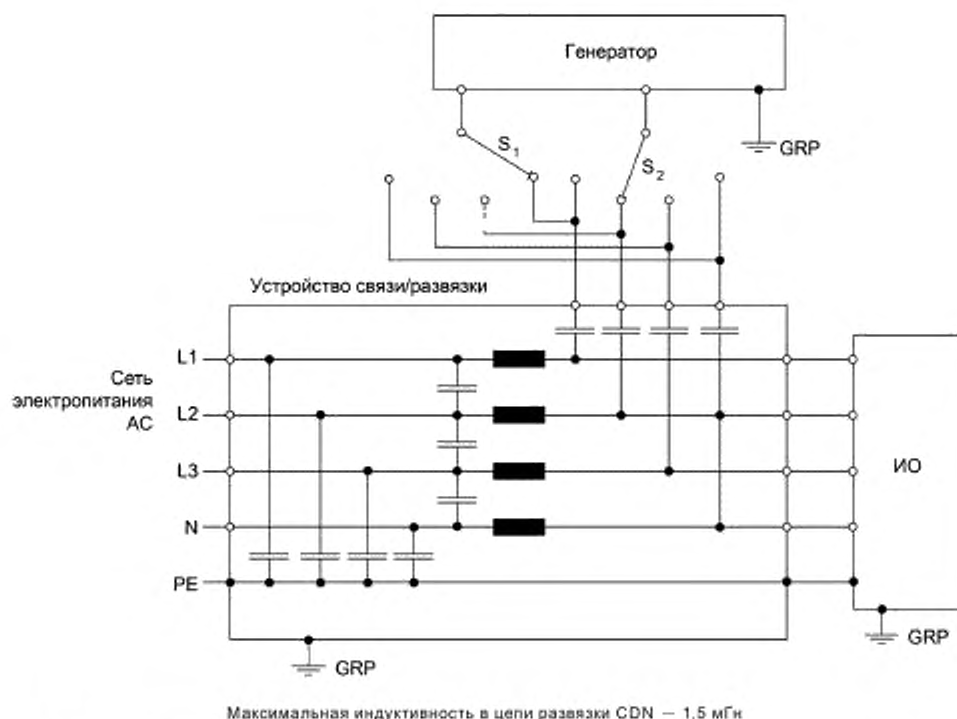
Рисунок 10a — Испытательная установка, снабженная опорной пластиной заземления (GRP)
