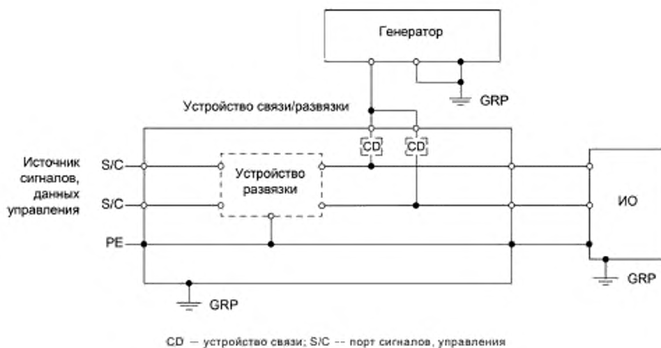
Рисунок 7a — Испытательная установка, снабженная опорной пластиной заземления (GRP)
