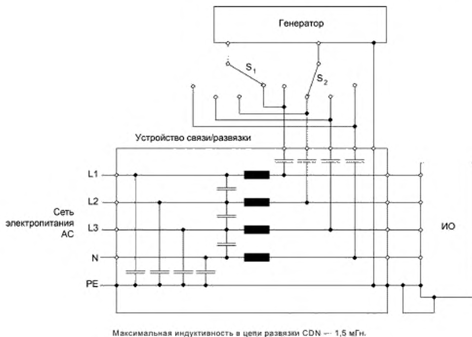
Рисунок 10b — Испытательная установка, снабженная специальными заземляющими проводниками
