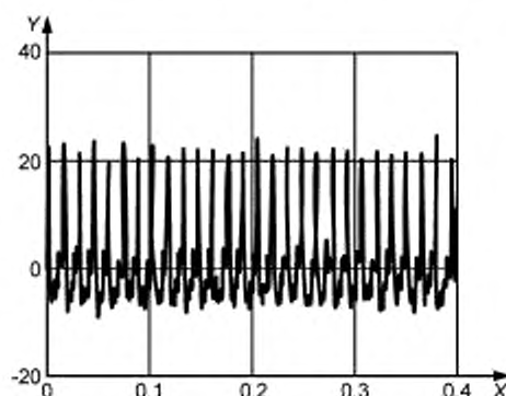
Рисунок В.5 — Временной сигнал при несоосности валов ([2])
