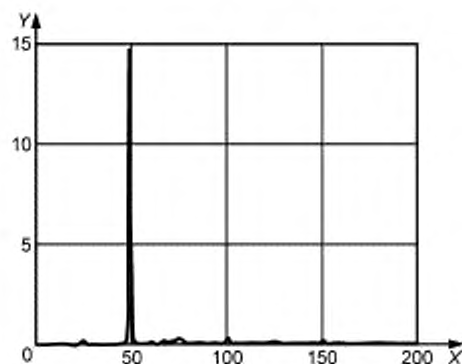
Рисунок В.6 — Вид спектра при повышенных механических напряжениях в присоединенном трубопроводе ([2])
