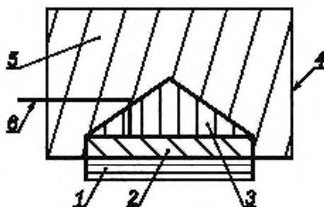
1 — пьезопластинка; 2 — контактный слой; 3 — механический демпфер; 4 — металлический экран; 5 — компауд; 6 — высокочастотный кабель
