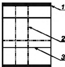
1 — электроды полуфабриката, полученные путем вжигания серебра; 2 — направление поляризации; 3 — направление разрезки
