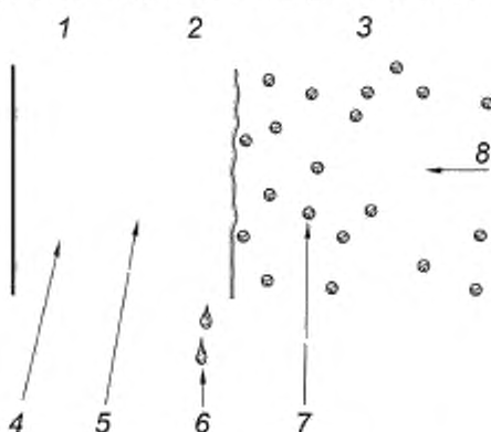
1 — лед; 2 — водяная пленка; 3 — холодный воздух; 4 — лед; 5 — жидкая вода; 6 — вытекающая вода; 7 — капли; 8 — направление ветра
