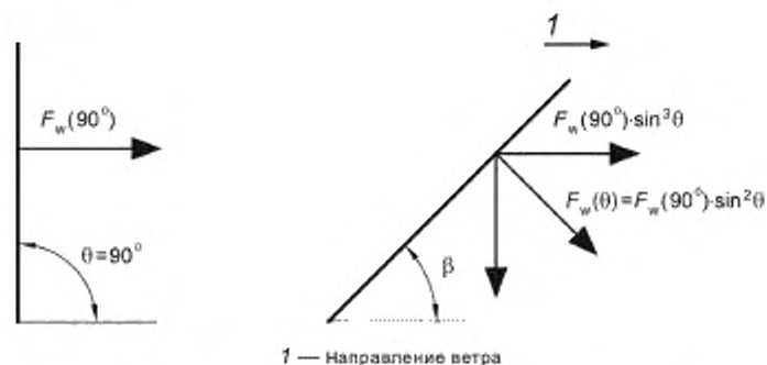
Рисунок 7 — Силы, действующие на наклонный элемент
