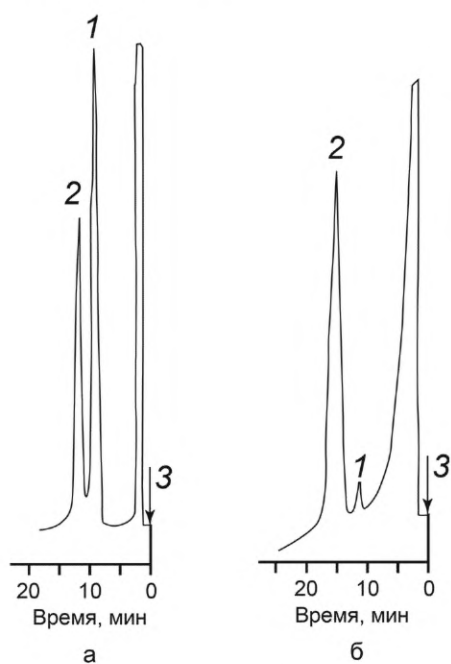
1 — фенол; 2 — м-крезол; 3 — ввод пробы
