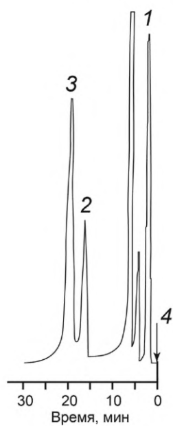
1 — ацетон; 2 — фенол; 3 — м-крезол; 4 — ввод пробы
