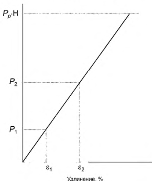
Рисунок 1 — Диаграмма нагружения
