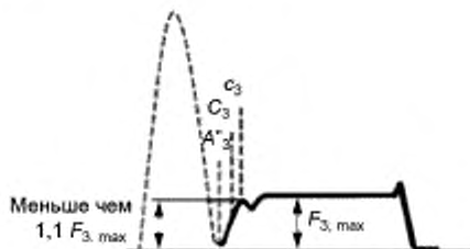
б) Экструдирование действующей силы наблюдается немедленно, после начала смачивания (до значения меньше, чем 1,1 F_{3,max} )
