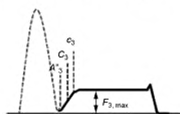
а) Смачивание начинается немедленно
