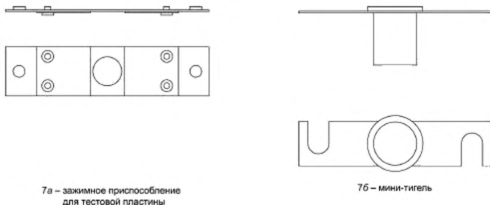
Рисунок 7 — Пример синхронного крепежа
