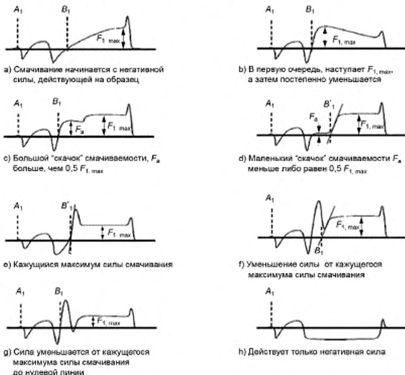
Рисунок В.1 — Типичные изменения силы смачивания в испытании с использованием метода быстрого нагрева
