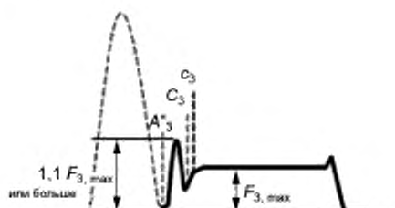
с) Экструдирование действующей силы наблюдается немедленно, после начала смачивания (до значения не менее 1,1 F_{3,max} )
