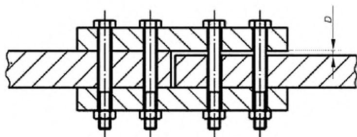
D -- зазор
