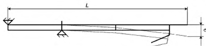
Рисунок 2 — Схема измерения прогиба штанги
