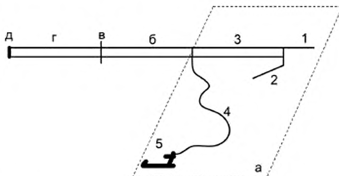
а — рабочая часть; б — изолирующее звено; в — ограничительное кольцо; г — рукоятка; д — заглушка; 1 — усовик; 2 — головки штанги; 3 — токопроводящее звено; 4 — заземляющий проводник по ГОСТ Р 57077; 5 — контактное соединение для крепления с рельсом по ГОСТ Р 57077
