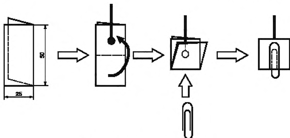
Рисунок 3 — Установка испытуемого образца
