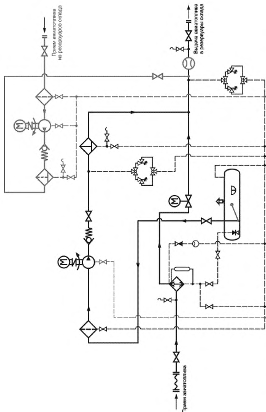
Рисунок Б.3 — Прием авиатоплива из танков нефтеналивных судов, стоящих на рейде, с гидропорожением шланговыми устройствами
