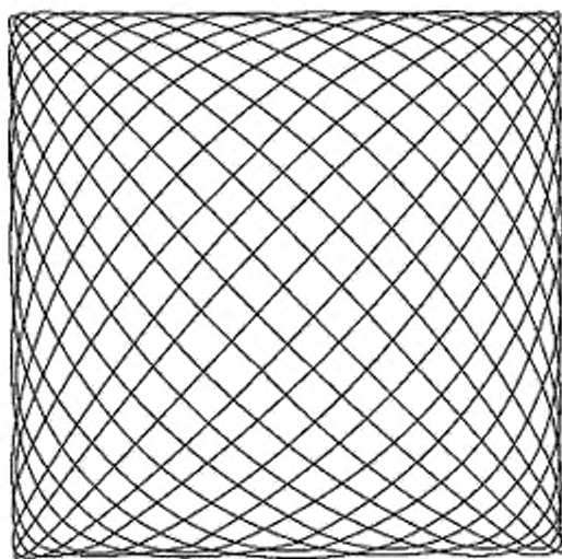
Рисунок 1 — Фигура Лиссажу
