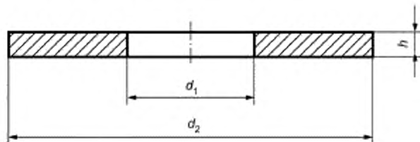
Рисунок 1 — Размеры
