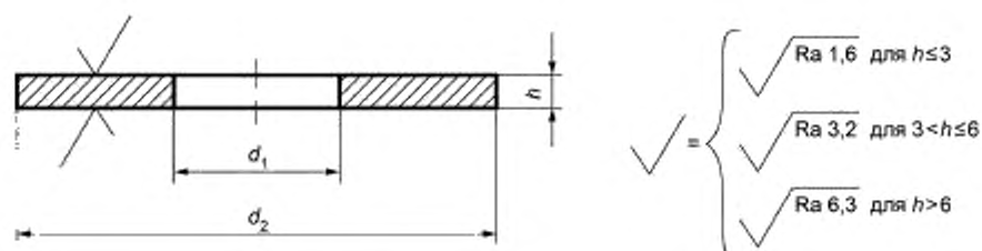
Рисунок 1 — Размеры
