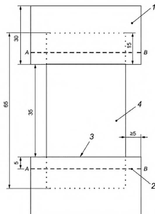
1 — ткань с покрытием, 2 — прошивка; 3 — линия, прочерченная на эластичном материале; 4 — эластичный материал
