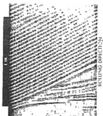
Рисунок А.19 — Линии скольжения (Людерса)
