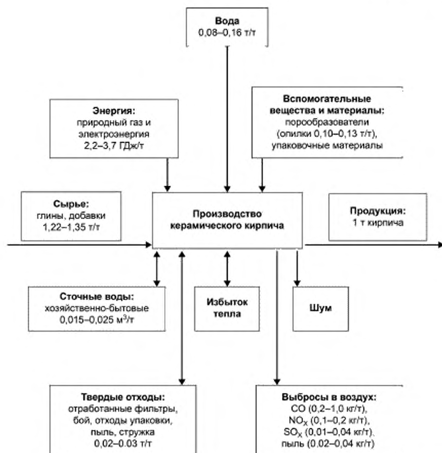
Рисунок А.1 — Входные и выходные потоки в производстве керамического кирпича в Российской Федерации (количественная оценка)
