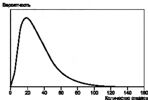
Рисунок С.3 — Субъективное распределение количества отказов
