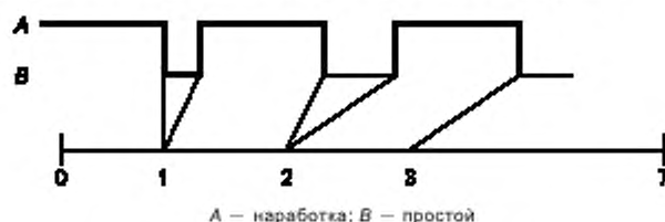
Рисунок 1 — Один восстанавливаемый объект
