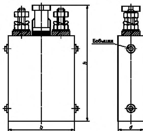
Рисунок 1 — Пример герметичного призматического аккумулятора в стальном корпусе с двумя выводами и четырьмя бобышками
