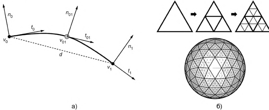
а) — обозначения, используемые для разбиения кривой; б) — треугольники разделены рекурсивно в глубину до пяти Рисунок А.1 — Типы треугольников, используемых в сетке
