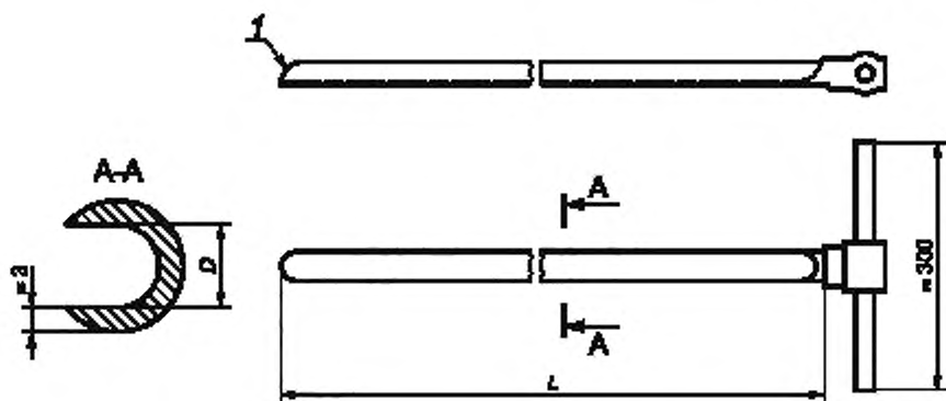
1 — острая кромка; D — внутренний диаметр; L — длина
