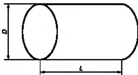
Рисунок 1 — Длина и диаметр пеллеты
