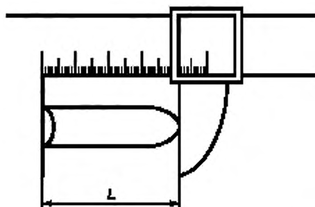
Рисунок 2 — Измерение штангенциркулем длины пеллеты между средней точкой выпуклости конца пеллеты и вогнутым поперечным сечением пеллеты
