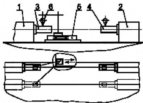
1 — передняя бабка; 2 — задняя бабка; 3, 4 — оправки; 5 — каретка; 6 — индикатор
