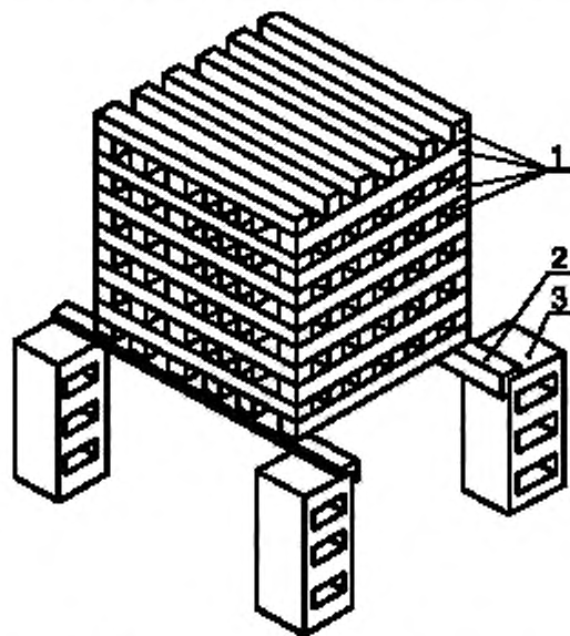
1 — деревянные бруски; 2 — стальной уголок; 3 — бетонный (металлический) блок
