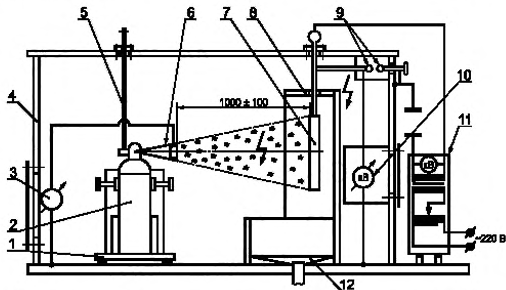
1 - изолирующая подставка; 2 - испытываемый огнетушитель; 3 - измеритель тока утечки; 4 - защитный каркас испытательного стенда; 5 - устройство запуска огнетушителя; 6 - насадка огнетушителя с электропроводным элементом; 7 - мишень; 8 - экран; 9 - разрядник; 10 - киловольтметр; 11 - источник высокого напряжения; 12 - емкость для сбора отработанного ОТВ
