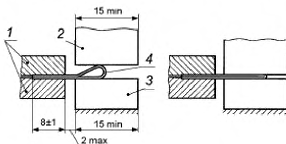
1 — зажим; 2 — пуансон; 3 — наковальня; 4 — образец
