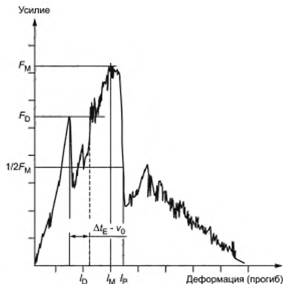
Первое повреждение (D) путем пробоа (P). \Delta t_E — время наступления первого повреждения на диаграмме «усилие — время». v_0 — скорость удара. F_M — максимальное усилие; t_M — деформация (прогиб) при максимальном усилии. t_P — деформация (прогиб) при пробоа
