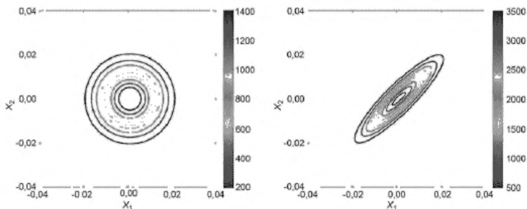
Рисунок 15 — Контурные линии совместных плотностей распределения входных величин в модели преобразования системы координат для примеров 1 (слева) и 4 (справа) (9.3.1.4)
