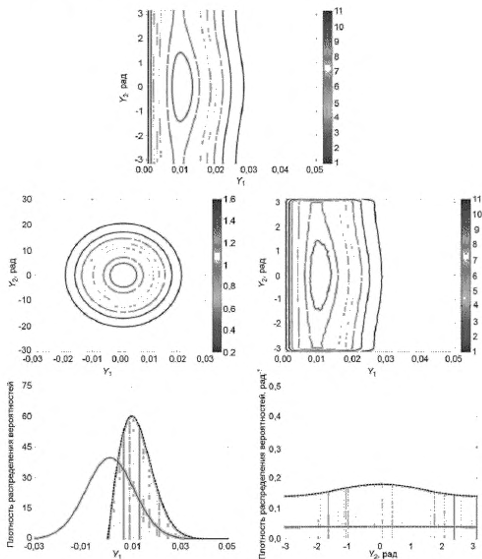
Рисунок 16 — Совместные плотности вероятности для Y , полученные аналитически (сверху), оценением по GUM (в центре слева) и методом Монте-Карло (в центре справа) и маргинальные плотности распределения для Y_1 (внизу слева) и Y_2 (внизу справа), полученные аналитически (пунктирная линия), оценением по GUM (сплошная линия) и методом Монте-Карло (гистограмма) для модели преобразования координат с x_1 = 0,001 и l(x_1, x_2) = 0 (9.3.2.2.2 и 9.3.2.2.3)
