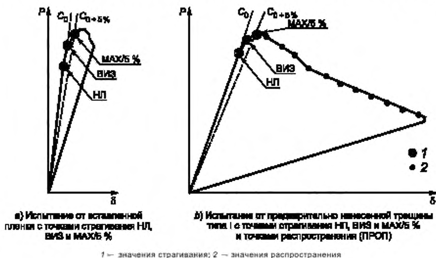
Рисунок 5 — График «нагрузка — смещение» для испытания образца ДКБ
