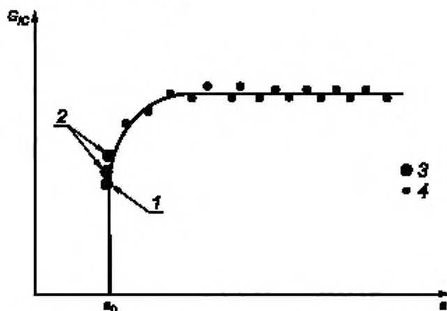
Рисунок 7 — Схематическая кривая сопротивления
