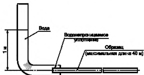
Рисунок 8 — Метод F5C, длинный образец
