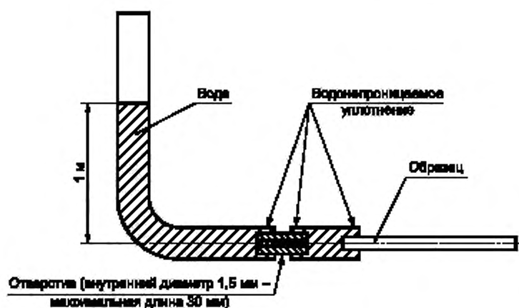
Рисунок 7 — Метод F5C, дюза
