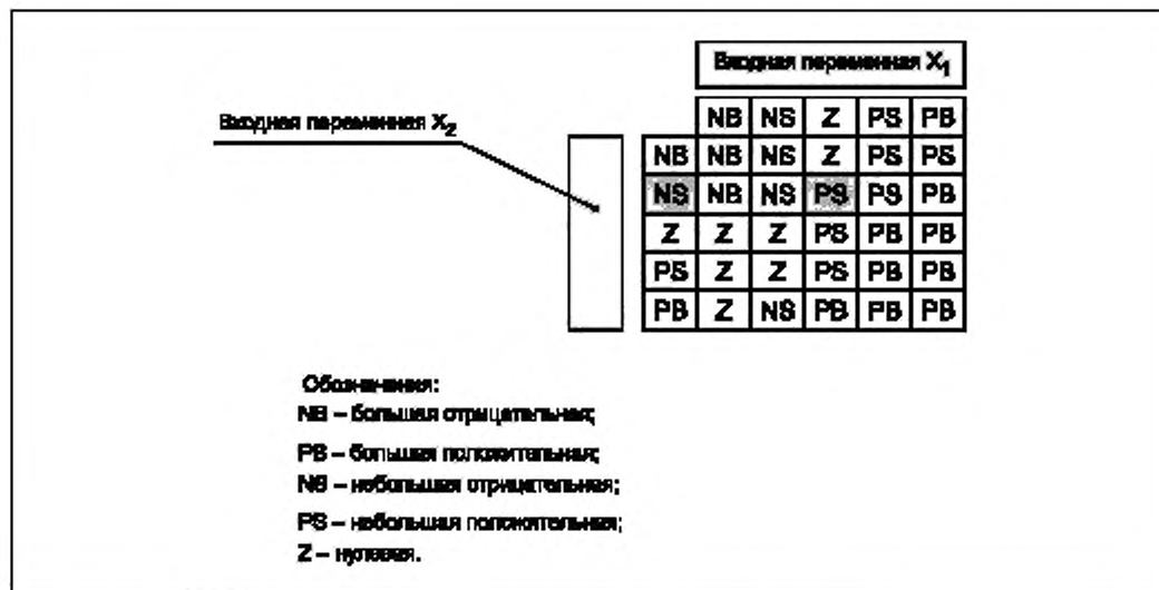
Рисунок А.8 — Матричное представление двух переменных
