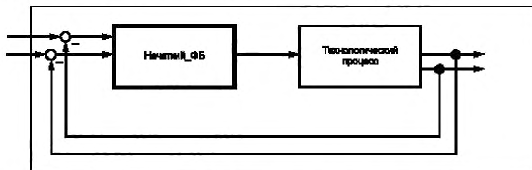
Рисунок В.3 — Пример прямого нечеткого управления
