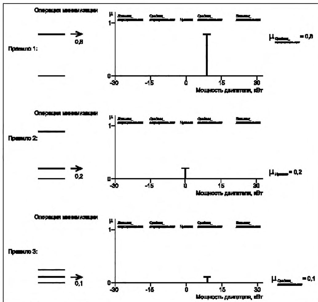
Рисунок С.12 — Принципы активации
