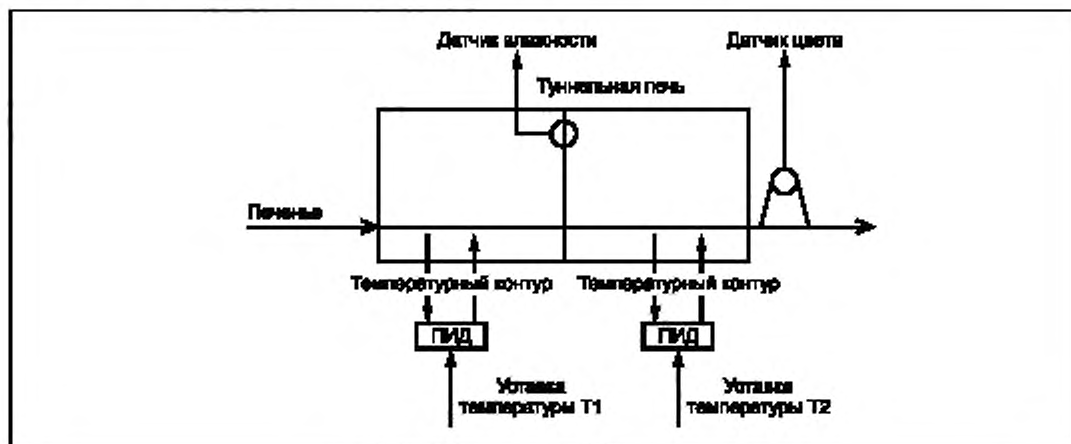
Рисунок D.1 — Принцип управления системой
