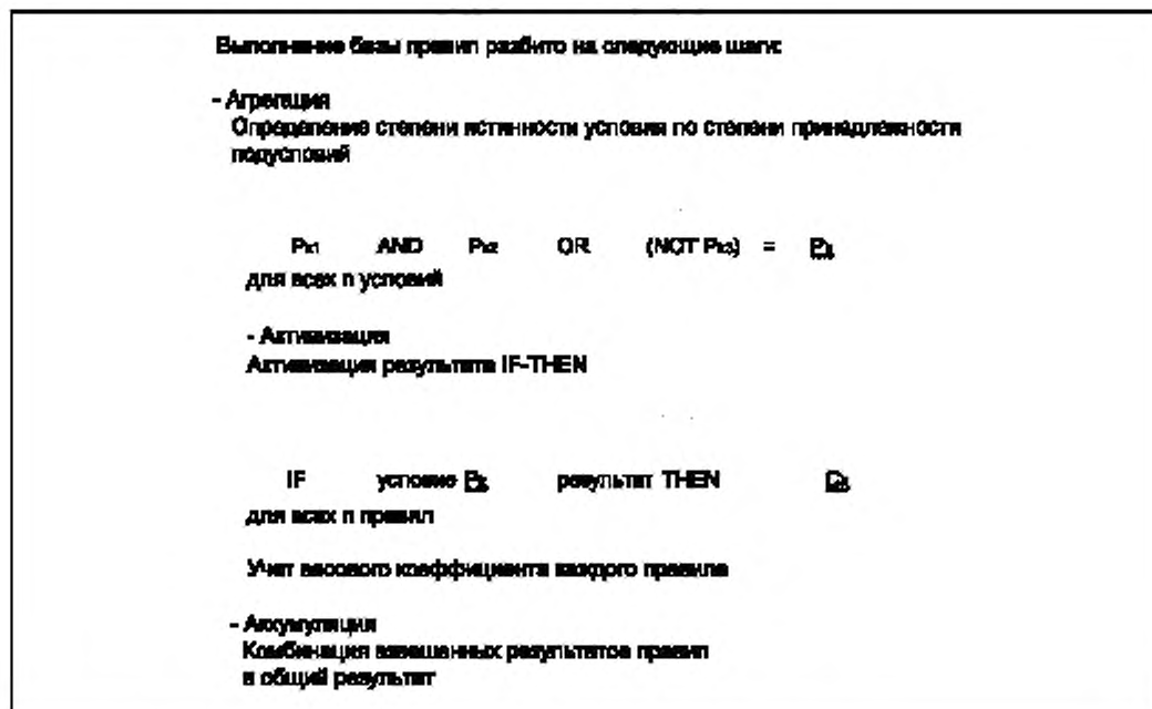
Рисунок А.9 — Элементы логического вывода
