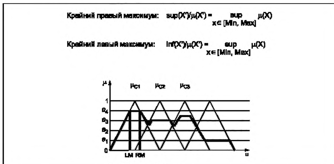
Рисунок А.11б — Разница между методами крайнего левого максимума и крайнего правого максимума
