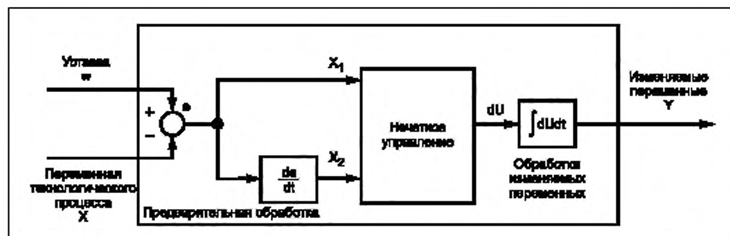
Рисунок А.13б — Пример основанного на нечетком управлении контроллера
