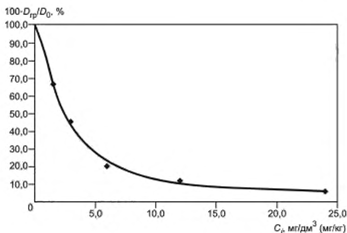
Рисунок 2 — Пример градуировочной характеристики для тест-системы № 2
