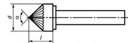
Рисунок 8 — Борфреза типов J и K
