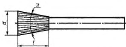
Рисунок 11 — Борфреза типа N
