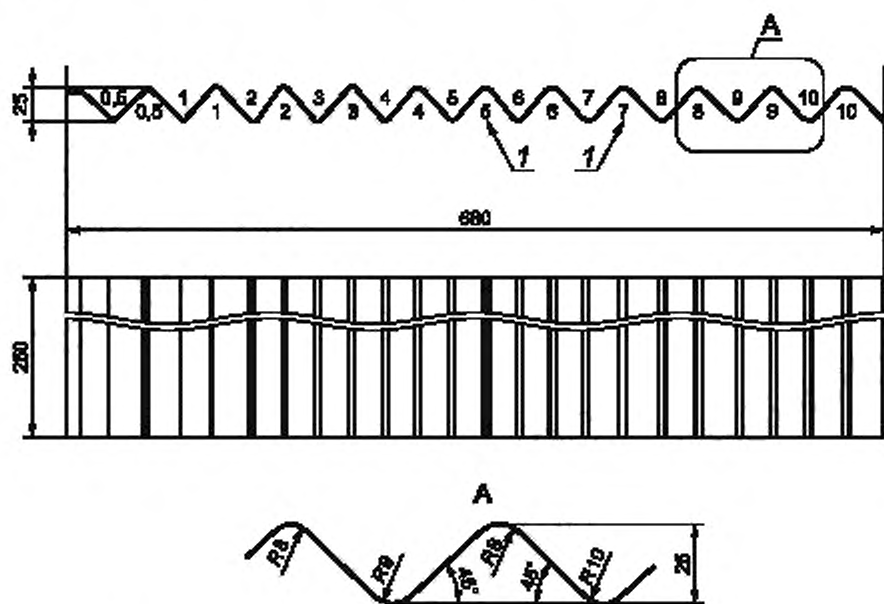
Рисунок 1 — Форма с изгибами переменного радиуса закругления
