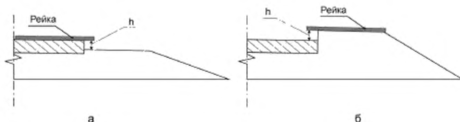
Рисунок 1 — Схема измерения величины занижения (возвышения) обочины и разделительной полосы: а — при занижении; б — при возвышении
