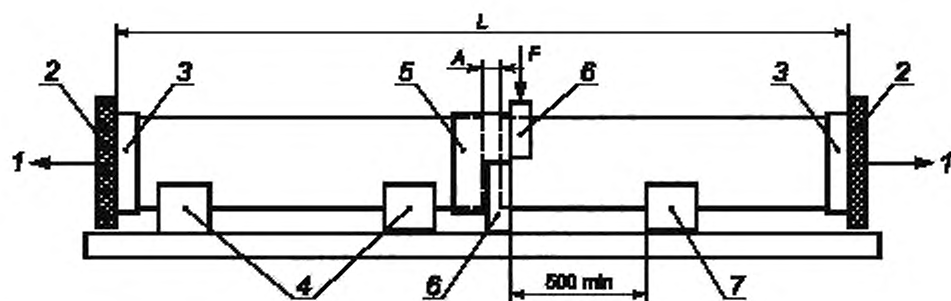
1 — осевое давление, действующее на образец для испытаний; 2 — оснастка испытательного стенда; 3 — торцевая заглушка; 4 — опоры; 5 — испытуемое соединение; 6 — хомут; 7 — опора «R»; A — общий вырыв, L — общая эффективная длина; F — сила смещения
