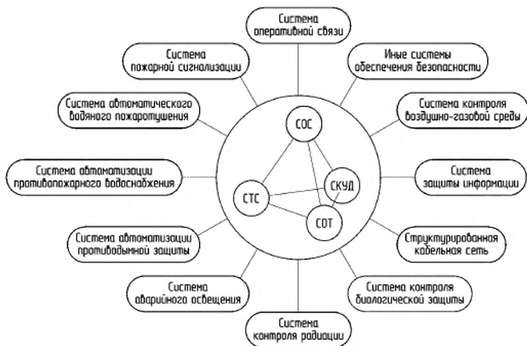
Функциональная схема ИСБ, составленная из базовых и иных вспомогательных и дополнительных систем
