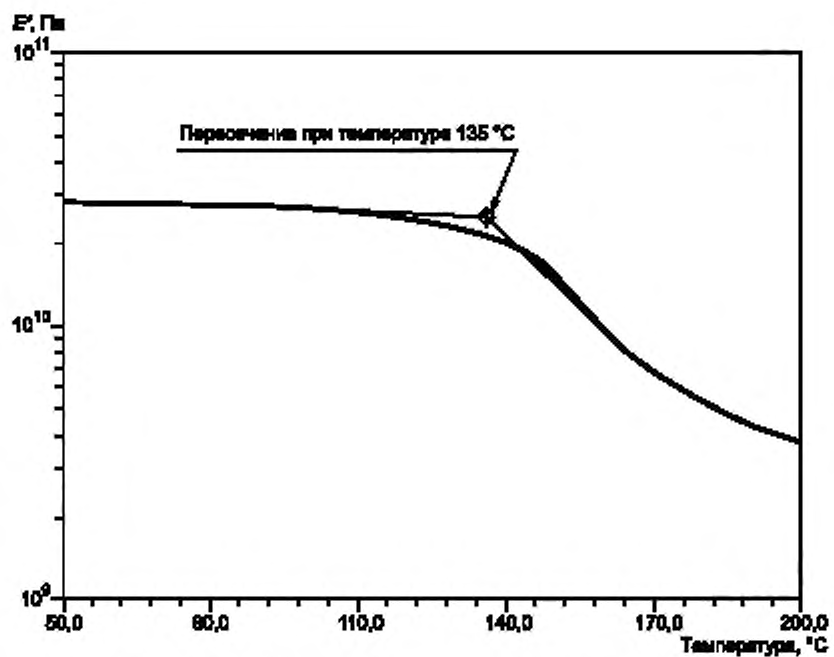
Рисунок X1.8 — Пример определения температуры стеклования T_g
