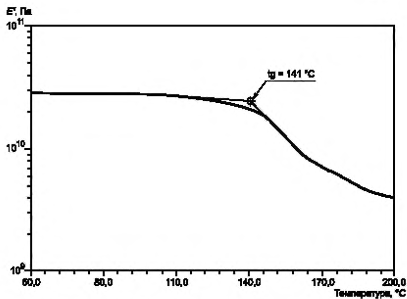
Рисунок X1.6 — Пример определения температуры стеклования T_g
