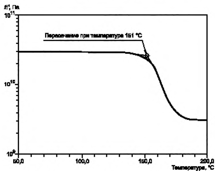
Рисунок X1.3 — Пример определения температуры стеклования T_g
