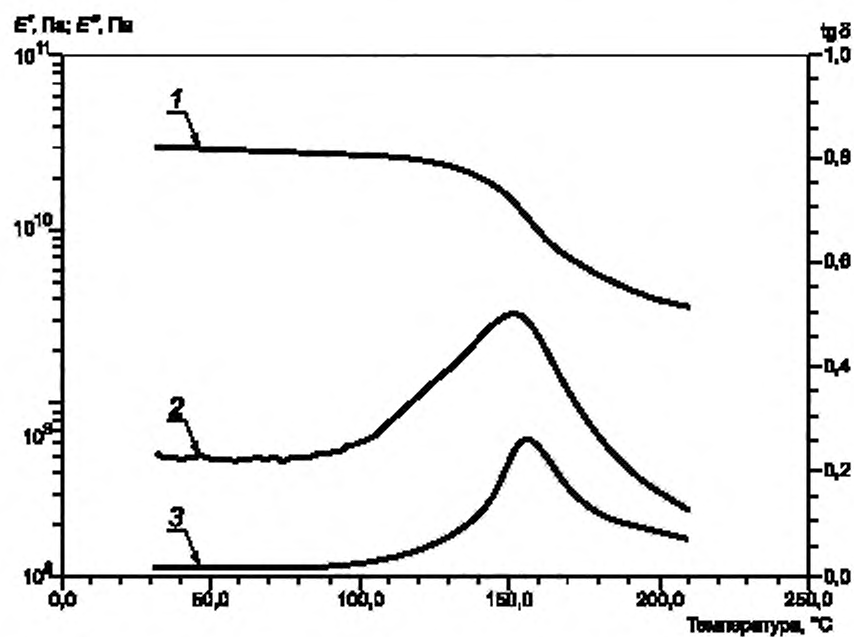
1 — график динамического модуля упругости E' ; 2 — график модуля потерь E'' ; 3 — график тангенса угла механических потерь \operatorname{tg} \delta
