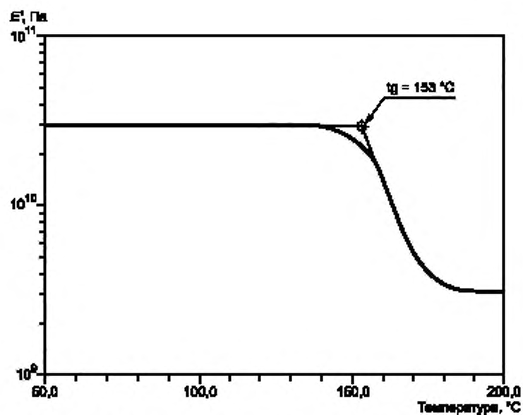
Рисунок X1.2 — Пример определения температуры стеклования T_g
