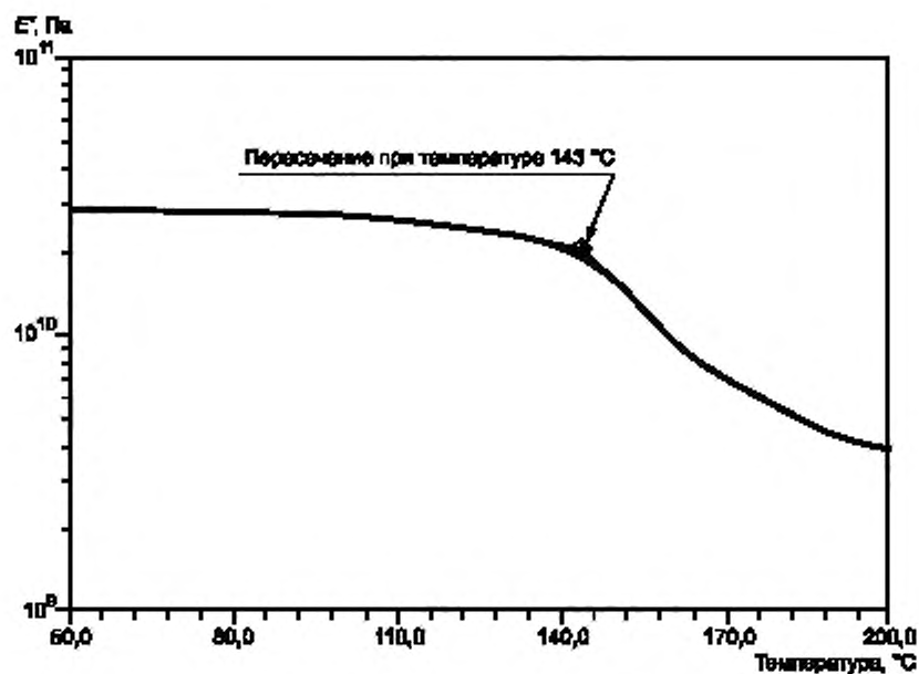
Рисунок X1.7 — Пример определения температуры стеклования T_g
