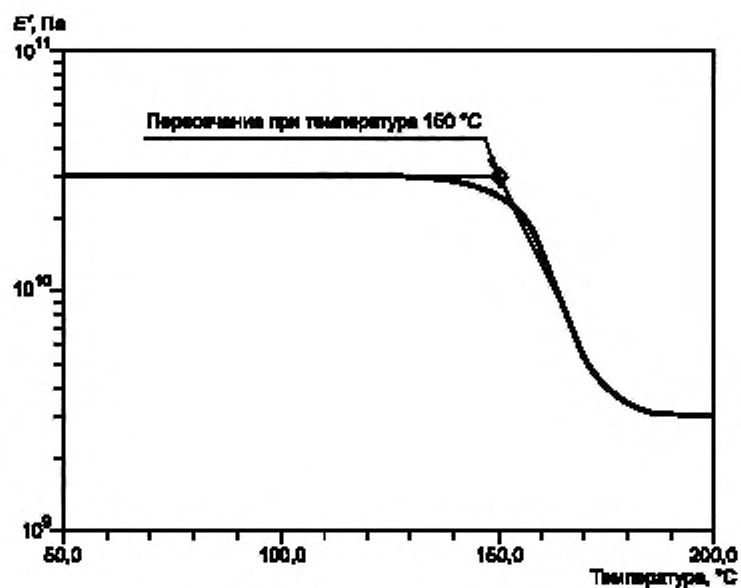
Рисунок X1.4 — Пример определения температуры стеклования T_g
