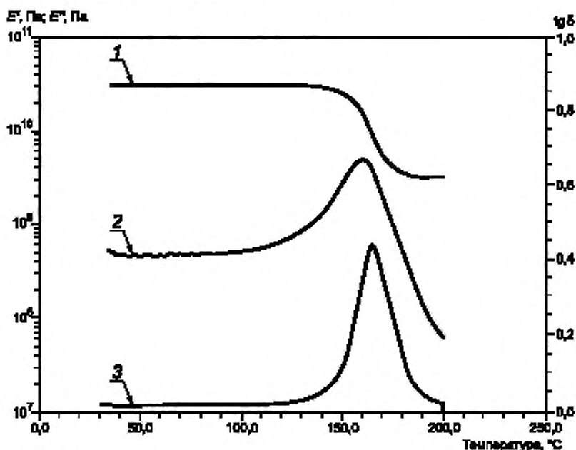
1 — график динамического модуля упругости E' ; 2 — график модуля потерь E'' ; 3 — график тангенса угла механических потерь \tan \delta
