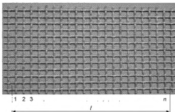
Рисунок 1 — Определение числа нитей
