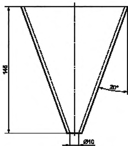
Рисунок 1 — Определение скорости растекания с помощью воронки
