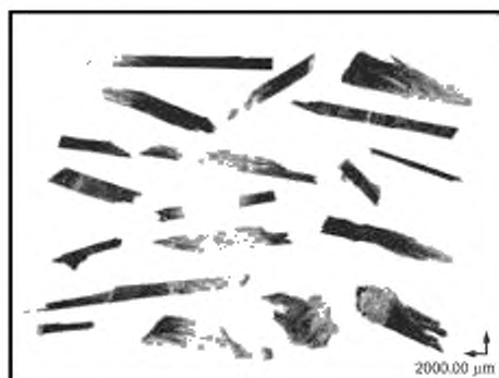
а — образцы измельченных полимерных композитов, армированных однонаправленным углеродным волокном
