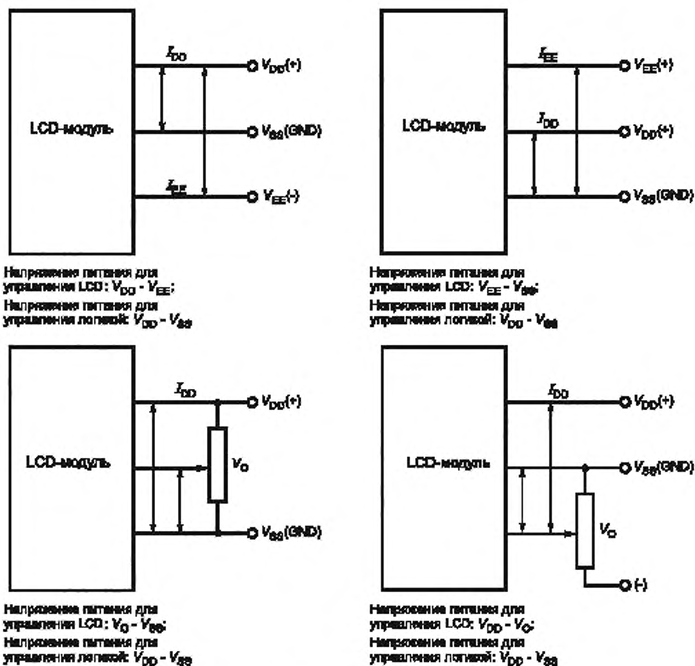
Рисунок 1 — Структурная схема для разъяснения подключения напряжения питания
