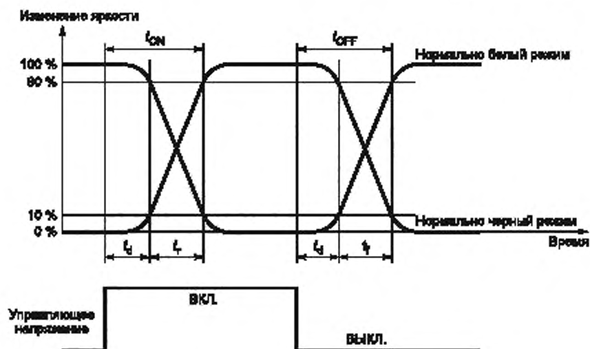
Рисунок 2 — Временная диаграмма для разъяснения времени отклика
