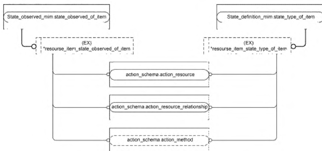
Рисунок D.8 — Представление ИММ на уровне объектов в формате EXPRESS-G. Диаграмма 7 из 7
