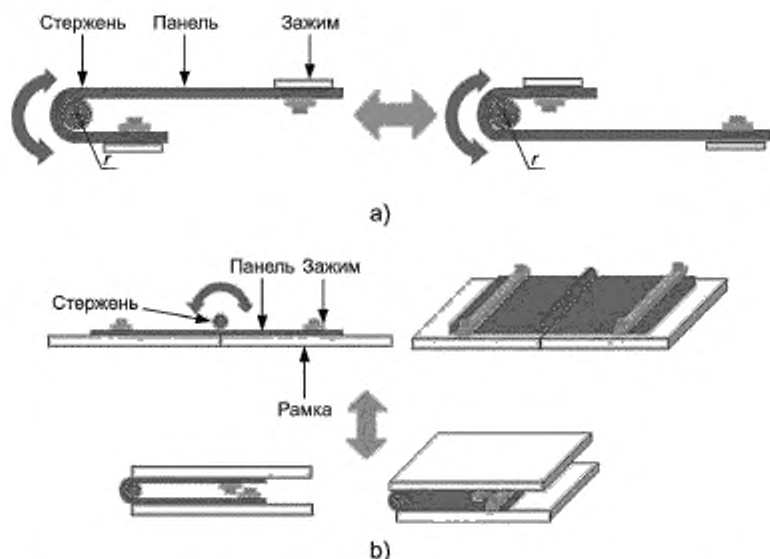
Рисунок 1 — Устройства для различных испытаний на циклический изгиб
