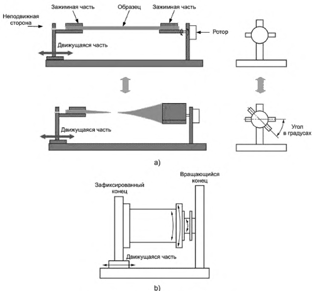
Рисунок 5 — Устройство для испытания на кручение
