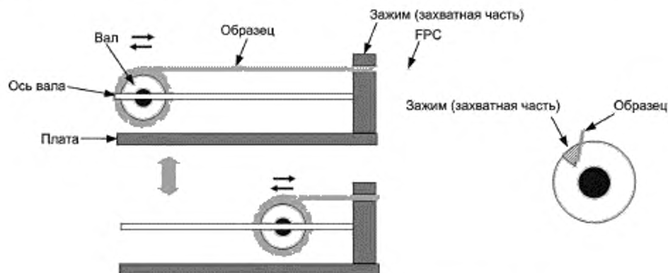
Рисунок 4 — Устройство для испытания на сворачивание (роллинг)
