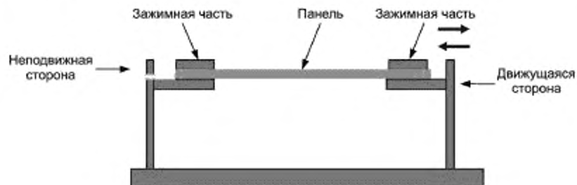
Рисунок 6 — Устройство для испытания на растяжение
