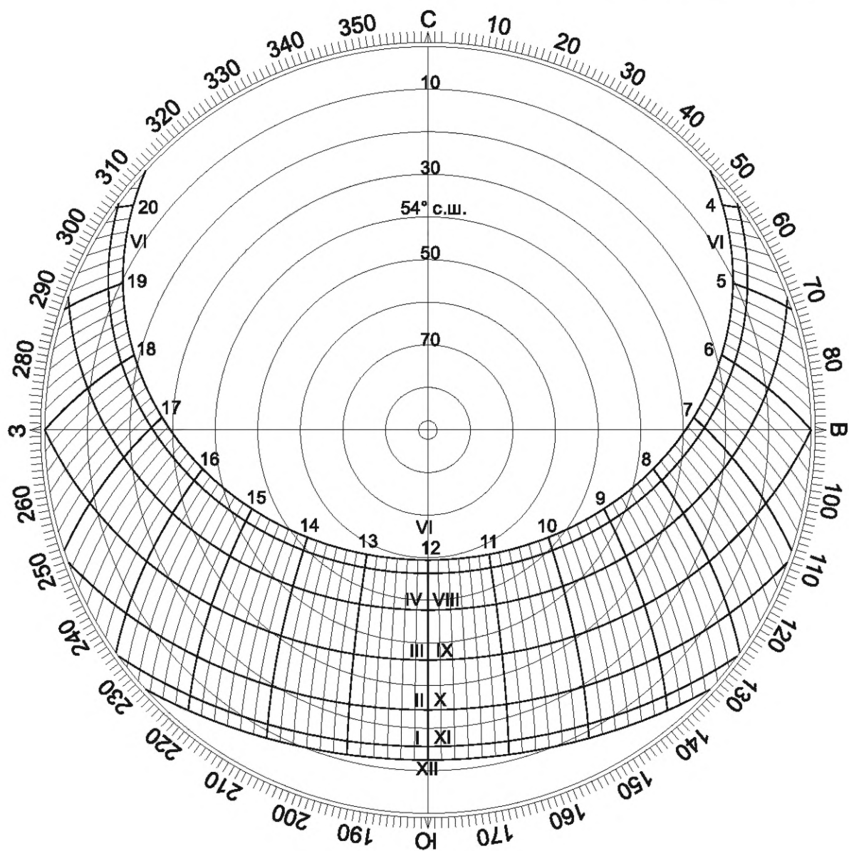
Рисунок Г.66 — Солнечная карта с равнопромежуточными альмукантаратами для территории Российской Федерации, расположенной на 54° с. ш.
