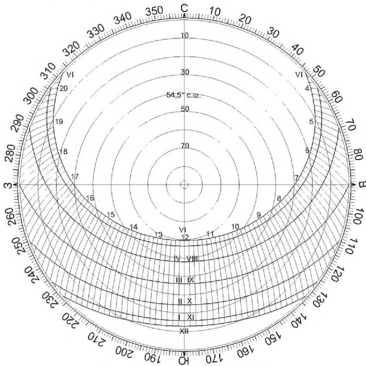
Рисунок Г.12 — Солнечная карта с равнопромежуточными альмукантаратами для города Москвы на 54,5^\circ с. ш.
