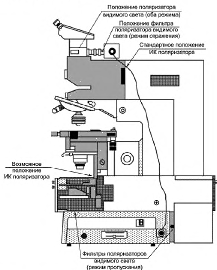
Рисунок 3 — Упрощенная схема приспособления для инфракрасной микроскопии
