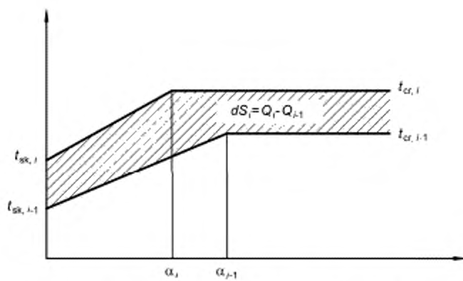
Рисунок А.2 — Распределение температуры в теле на моменты времени t_{sk,i-1} и t_{sk,i}
