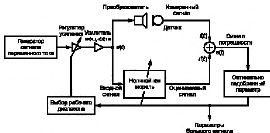
Рисунок 4 — Установка для динамического измерения параметров больших сигналов
