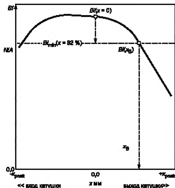
Рисунок 5 — Определение максимального пикового смещения x_D , ограниченного только коэффициентом силы
