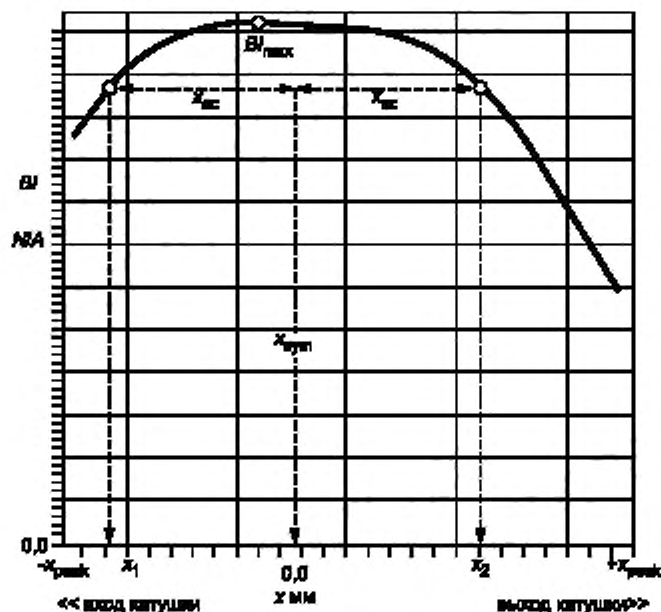
Рисунок 7 — Определение точки симметрии x_{\text{sym}} характеристики нелинейного коэффициента силы Bl(x)
