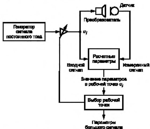
Рисунок 2 — Установка для статического и квазистатического измерений
